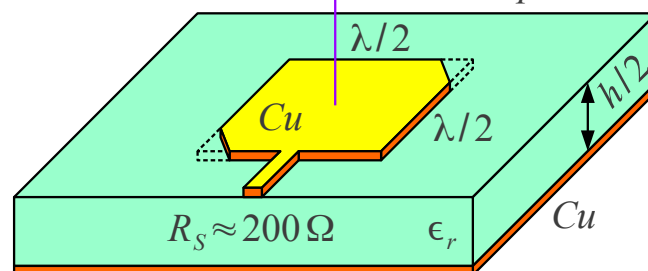
Obrezana mikrotrakasta krpica
