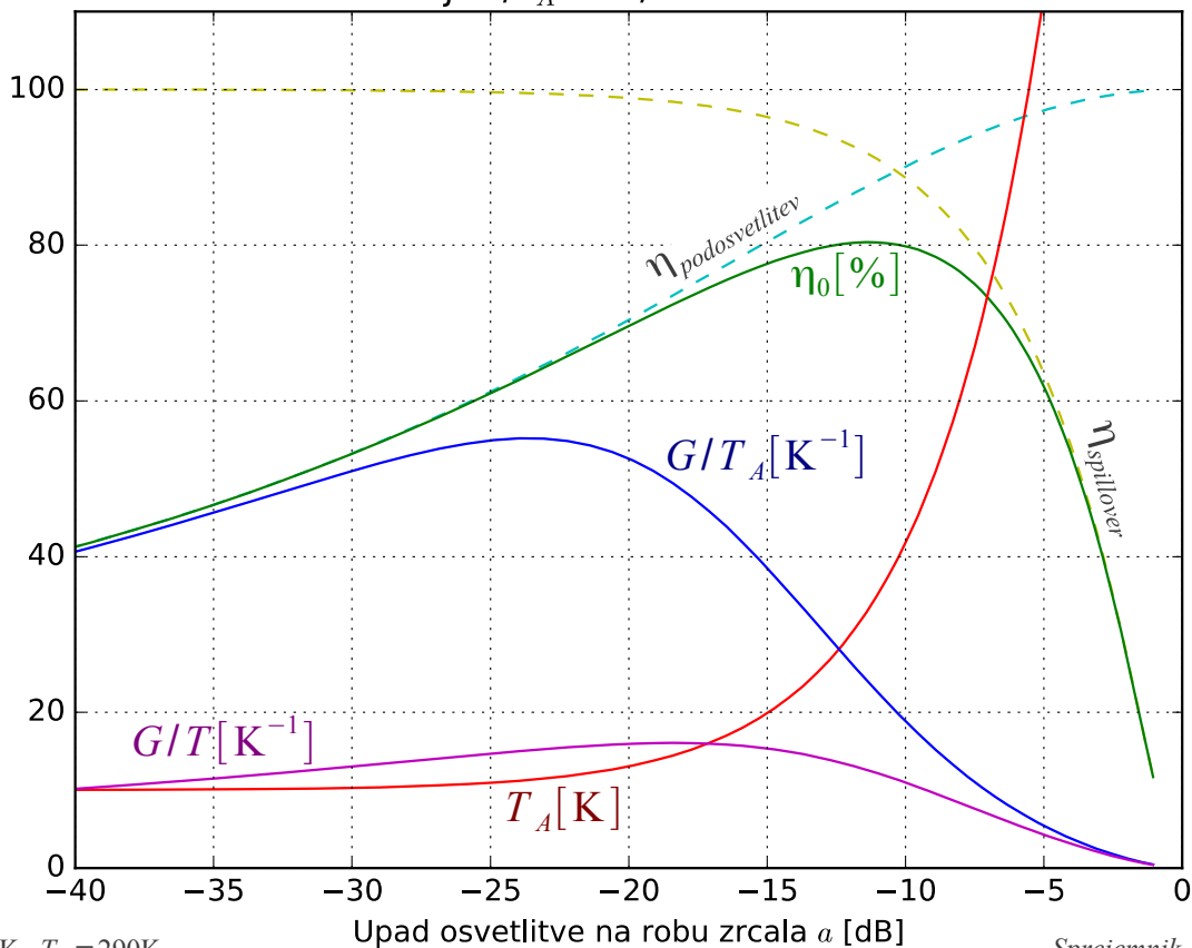
Razmerji G/T_A in G/T zrcalne antene
