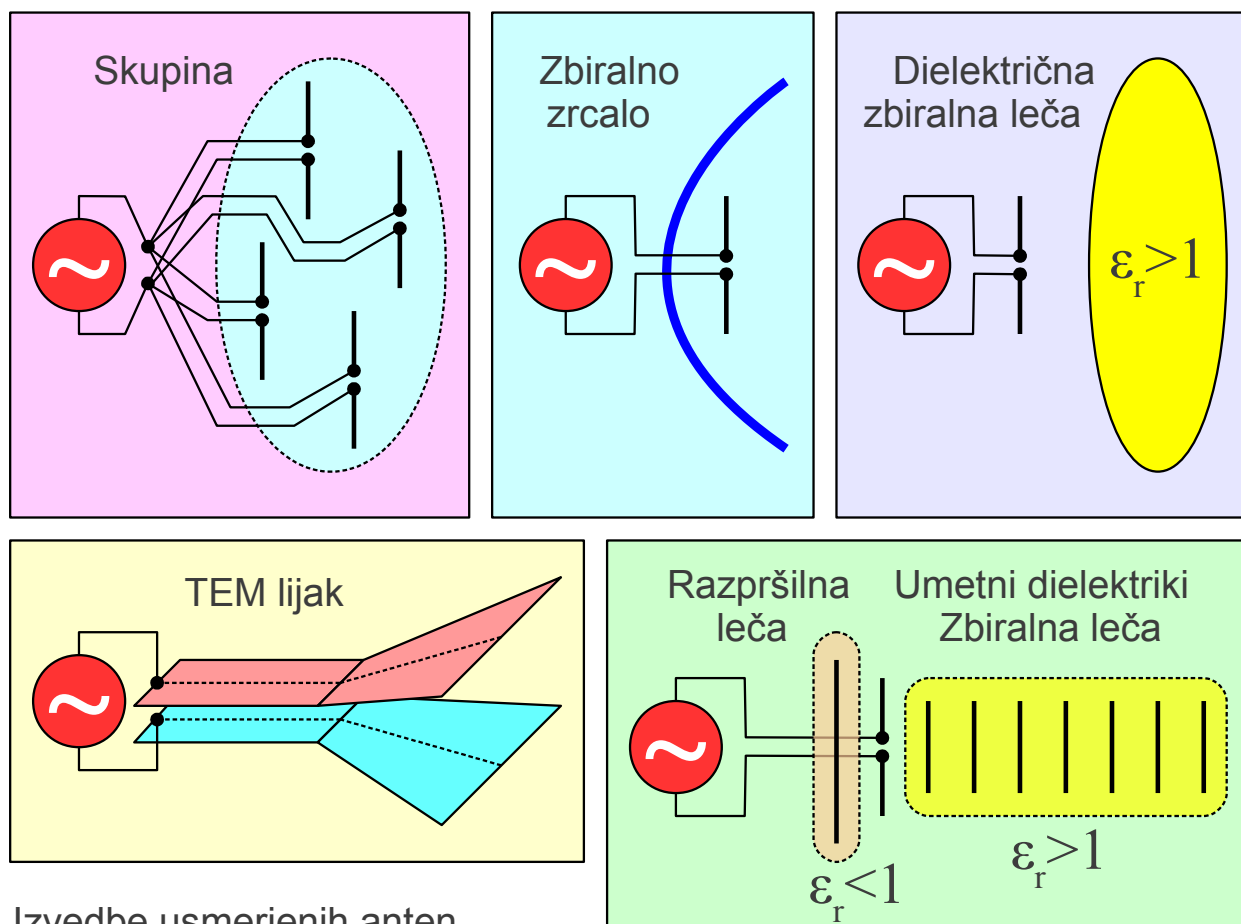
Izvedbe usmerjenih anten
