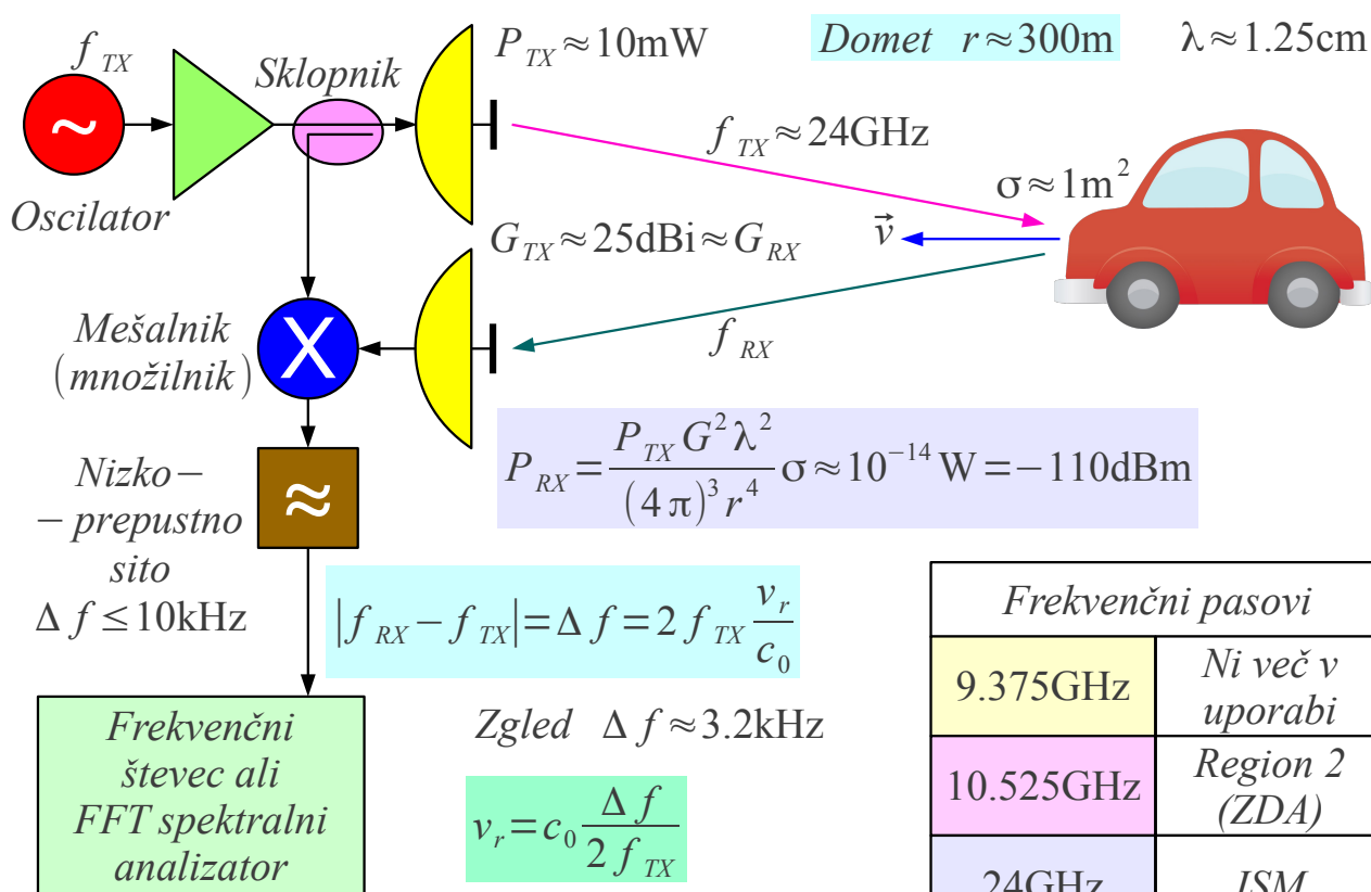
CW Dopplerjev radar
