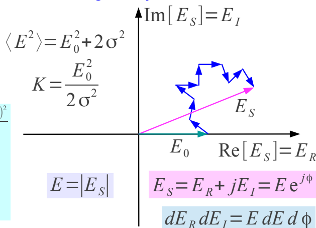
Večpotje z neposrednim žarkom: Rice ( E_0, \sigma ) en velik in mnogo naključnih malih kazalcev
