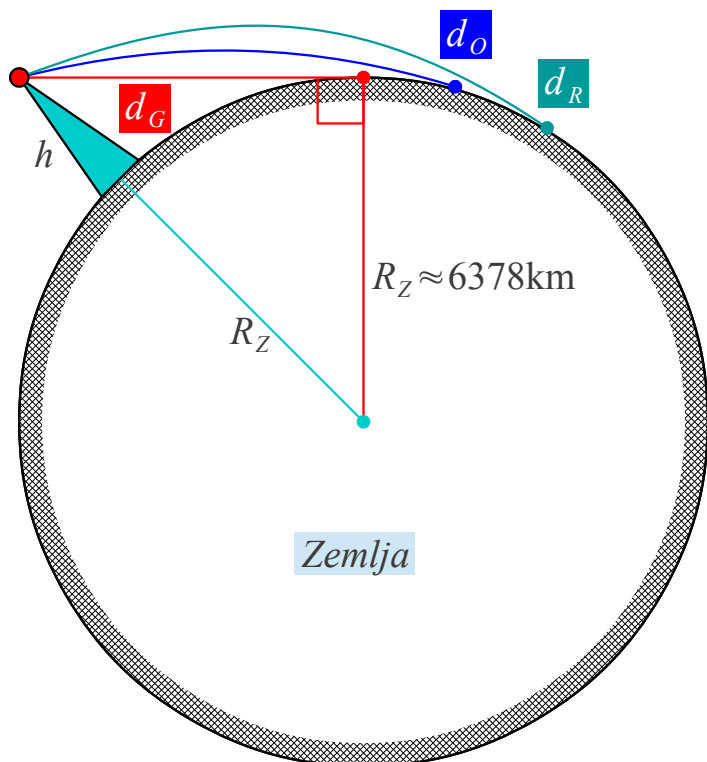
Geometrijska, optična in radijska vidljivost
