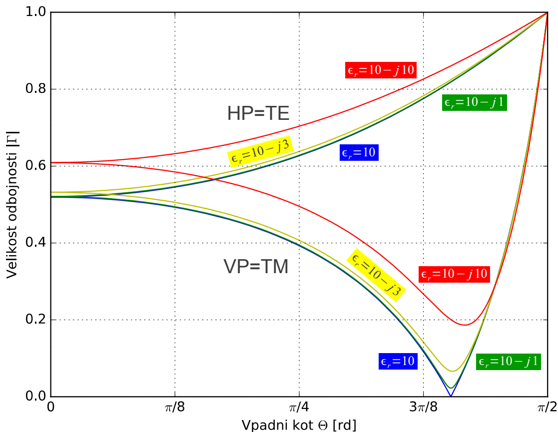
Dielektrik z izgubami \epsilon_r = 10, 10-j1, 10-j3, 10-j10
